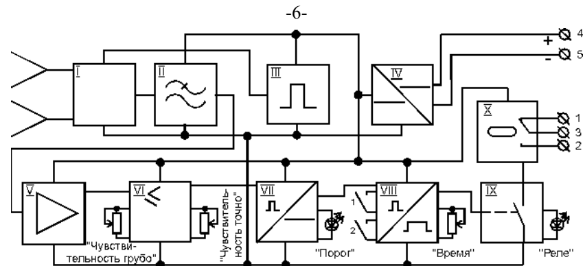
Рис. 3. Структурная схема РДД-02А.
