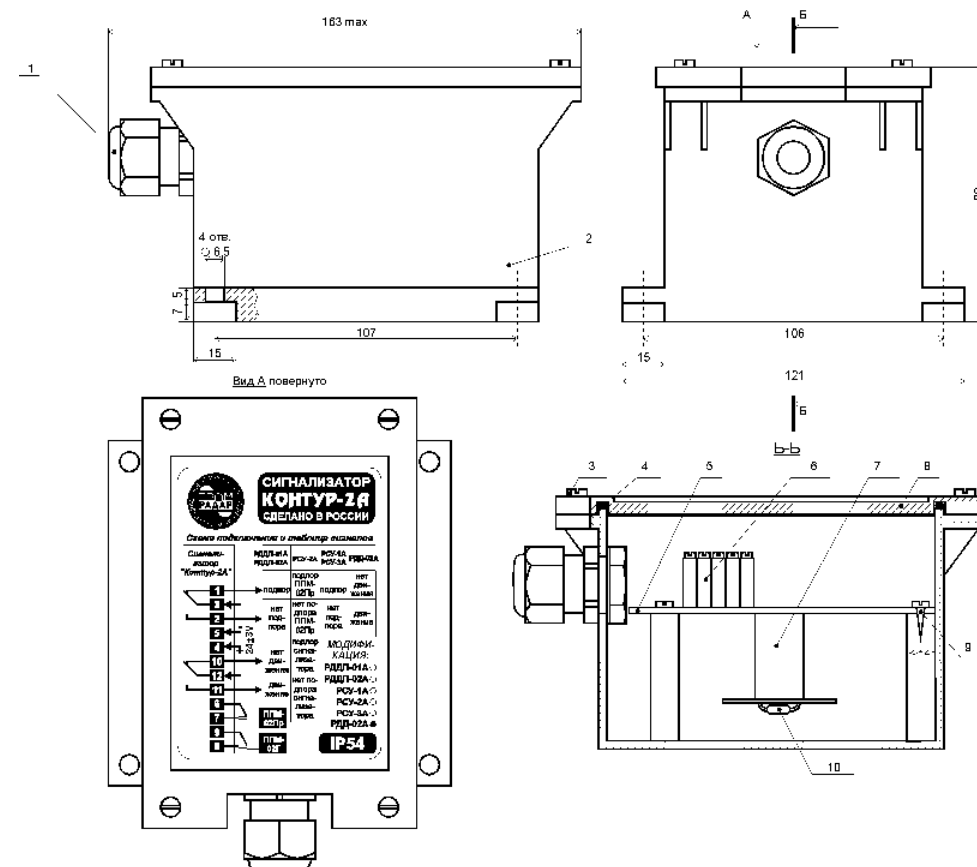
Рис. 1. Конструкция сигнализатора «Контур-2А» (модификация «РДД-02А»).
